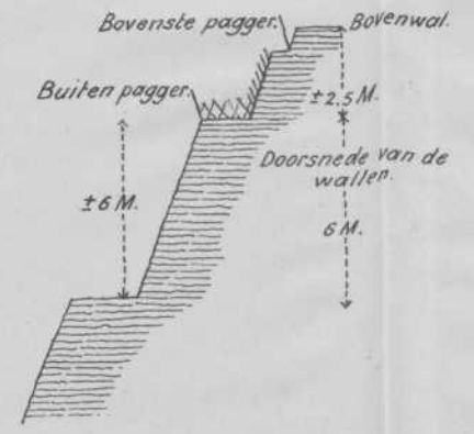
Fig. 4. Doorsnede op fig. 3.
